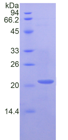
15% SDS-PAGE
